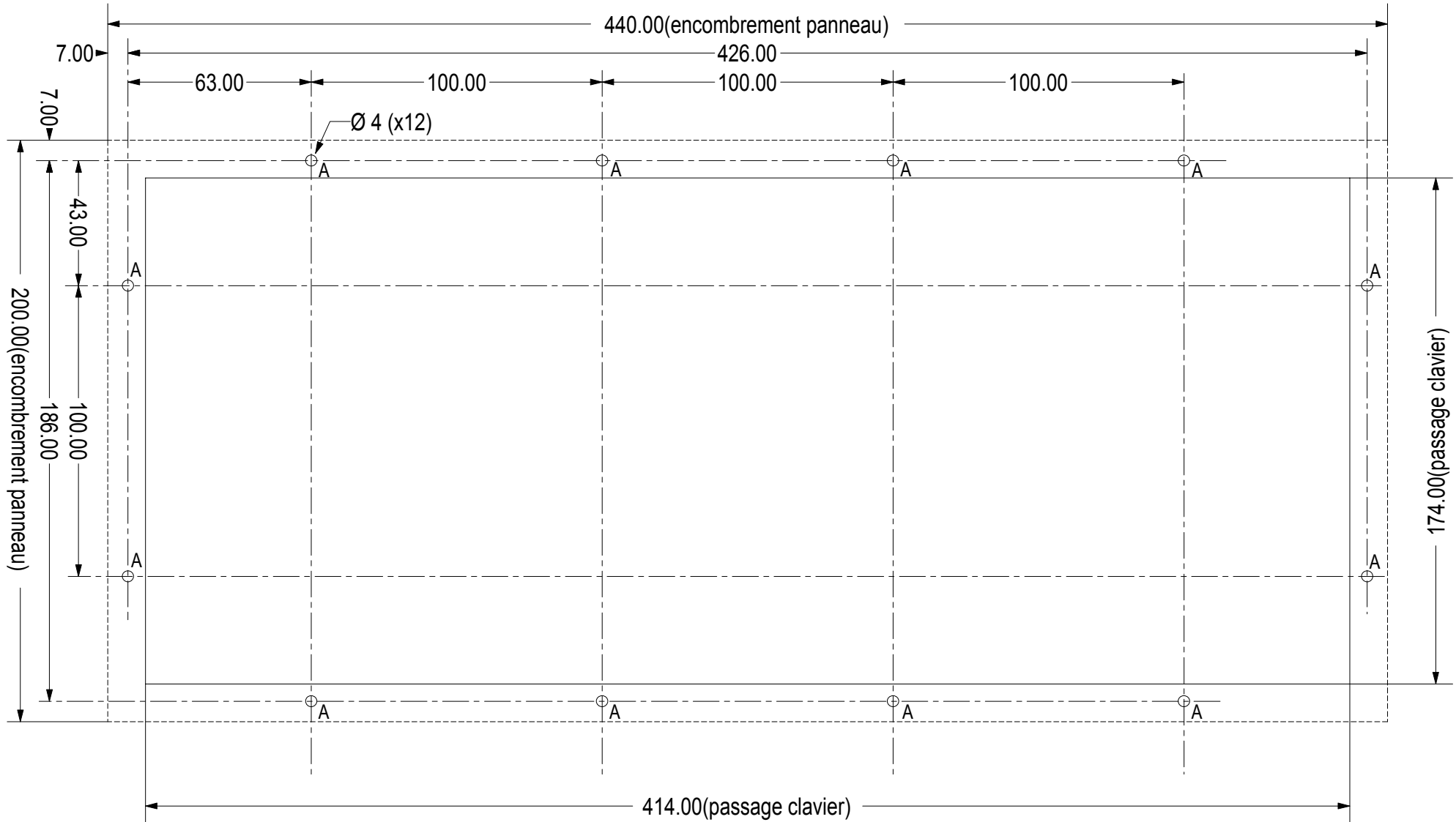
PLAN D'INTEGRATION DU CLAVIER NX-105TL-TB38-MODUL
