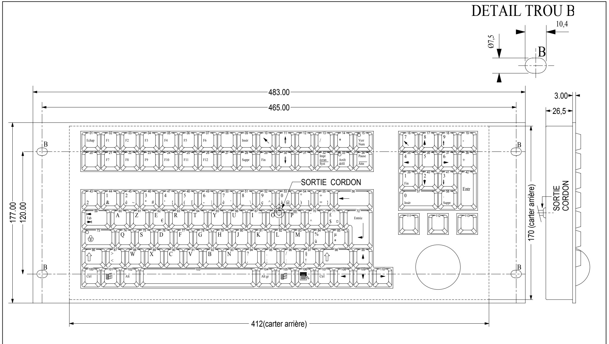
PLAN D'ENCOMBREMENT CLAVIER NX-105TL-TB38-FP
